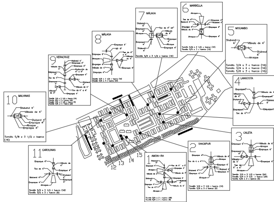
Fig.4 Detalles hidráulicos. Alcaldía Coyoacán.
