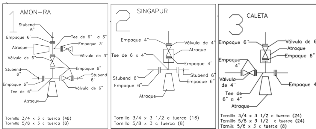
Fig.3 Detalles Hidráulicos de diversas calles de la Alcaldía Coyoacán.
