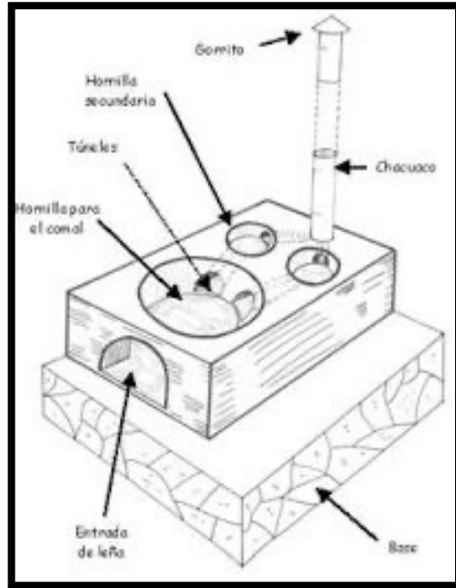
Imagen 5 "Ilustración de una estufa Lorena tradicional"
