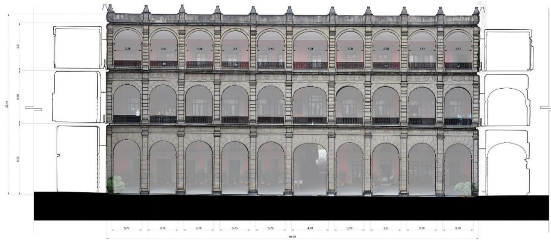
Larguillo + Plano Fachada Oriente Patio Central
