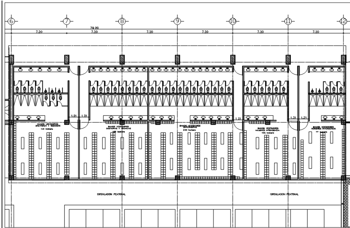
Fig. 1 Propuesta de distribución de núcleo de sanitarios del proyecto arquitectónico "Hospital General de Zona" No. 20 "Las Margaritas".
