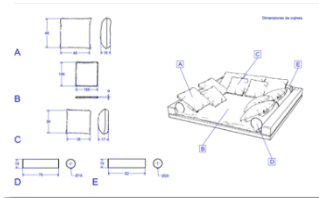
(Planos técnicos para fabricación.)
