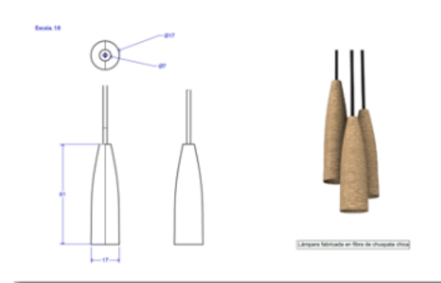
(Planos técnicos para fabricación.)
