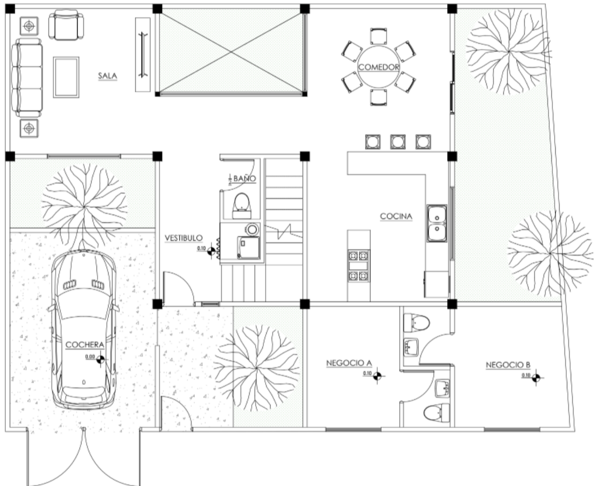
PLANTA BAJA ESC: 1:30
