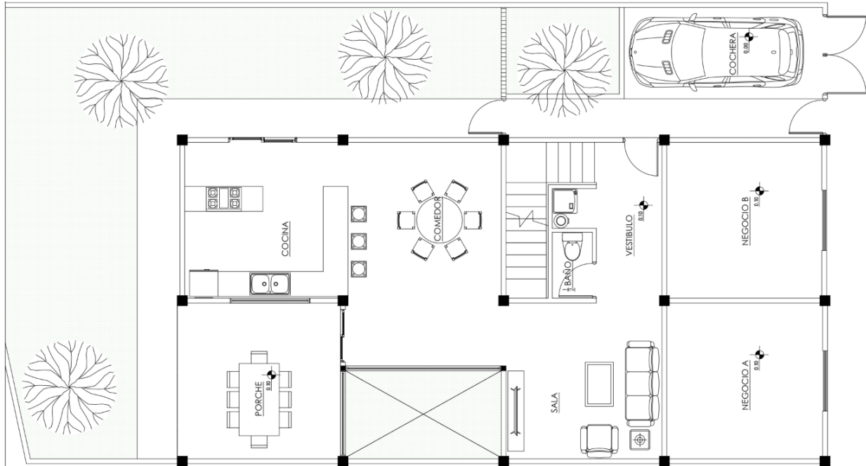
PLANTA BAJA ESC: 1:30
