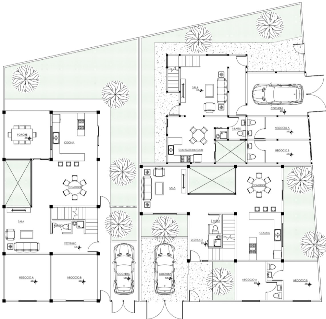
PLANTA DE CONJUNTO ESC: 1:50
