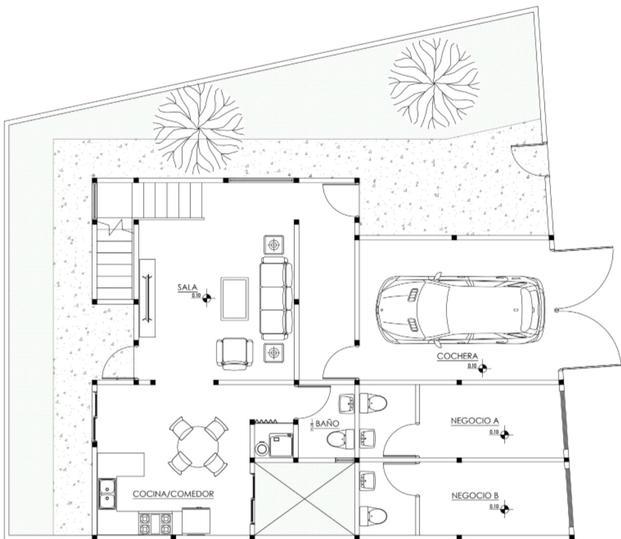
PLANTA BAJA ESC: 1:30
