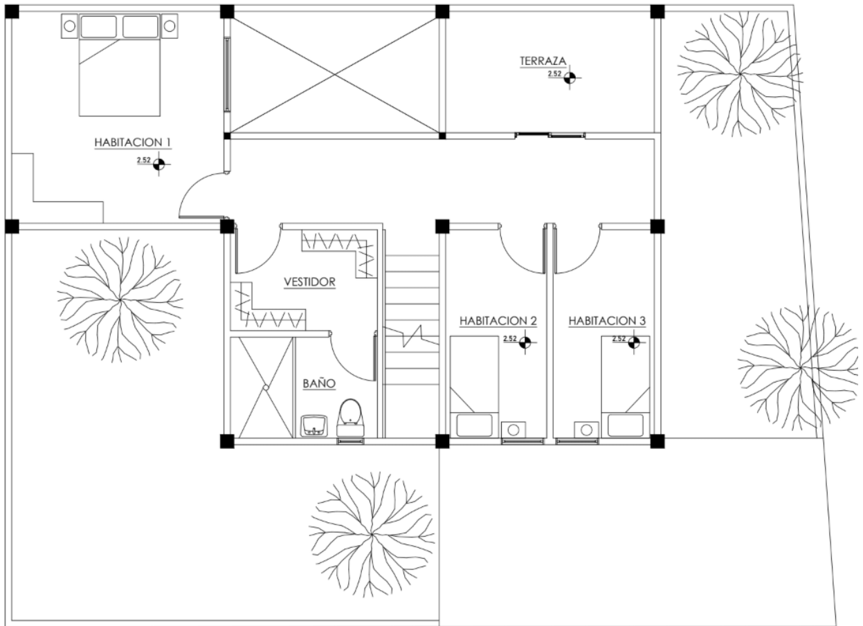
PLANTA ALTA ESC: 1:30
