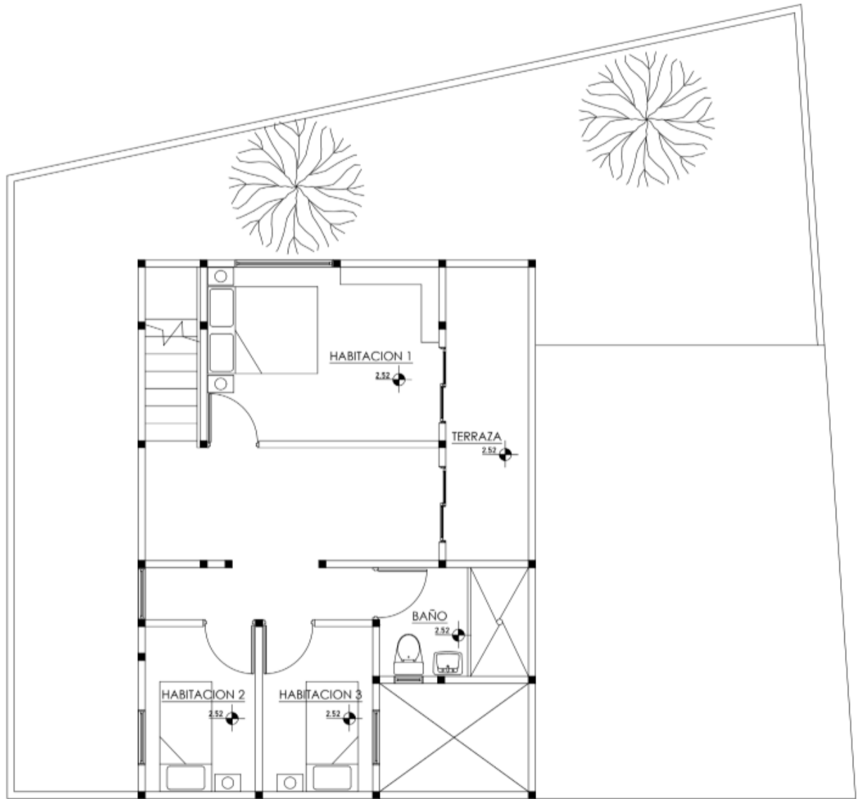
PLANTA ALTA ESC: 1:30
