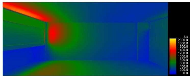
Asoleamiento Aula Edificio D 10:00 a.m.
