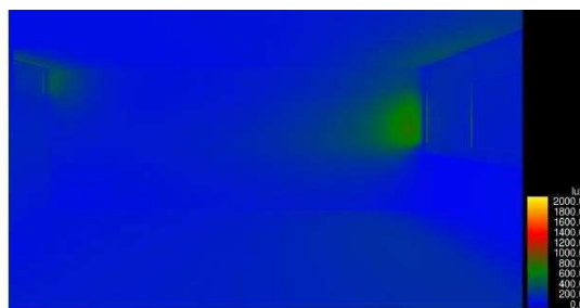
Asoleamiento Aula Edificio B 06:00 p.m.
