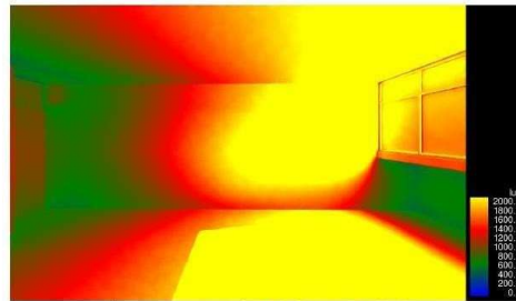
Asoleamiento Aula Edificio B 8:00 a.m.
