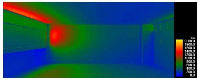
Asoleamiento Aula Edificio D 02:00 p.m.
