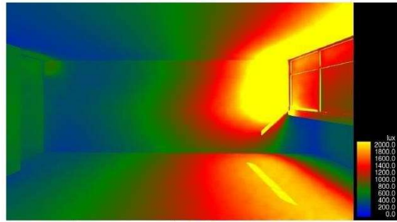
Asoleamiento Aula Edificio B 10:00 a.m.
