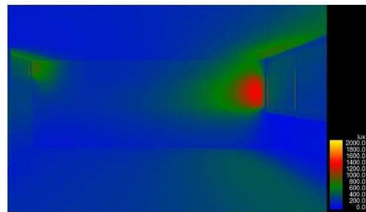
Asoleamiento Aula Edificio B 04:00 p.m.
