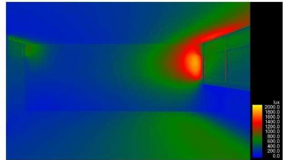
Asoleamiento Aula Edificio B 02:00 p.m.
