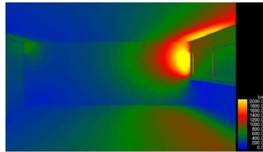
Asoleamiento Aula Edificio B 12:00 p.m.
