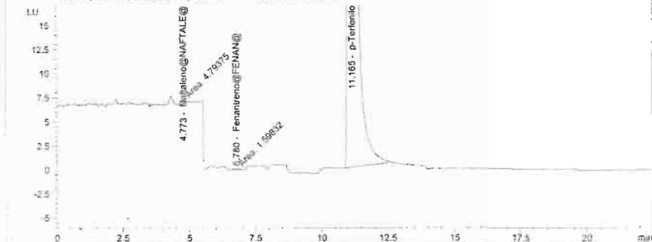
WVD1 A, Wavelength=230 nm, TT (MARZO2~1\0308538\538PAH35.D)
