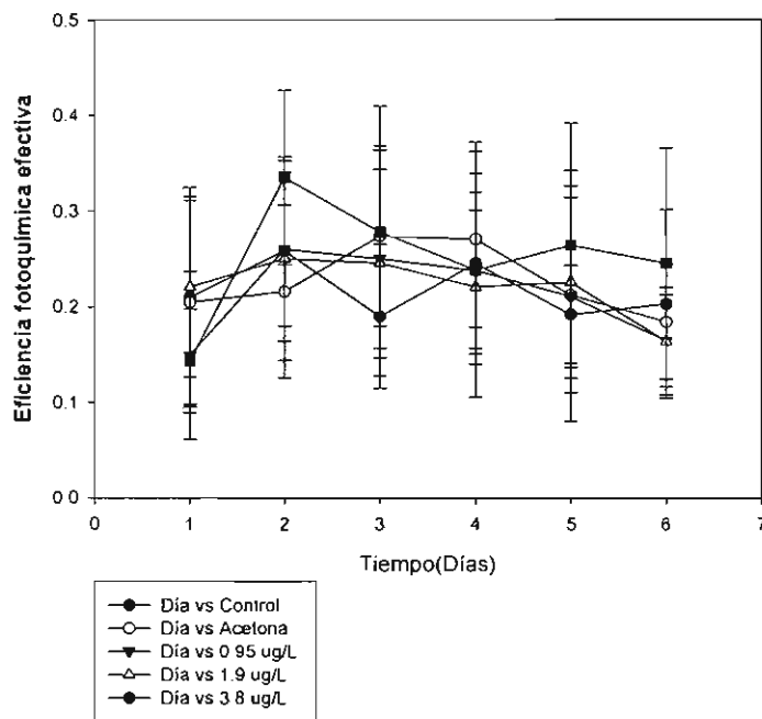
Figura 27. Eficiencia fotoquímica efectiva del coral Porites divaricata expuestos a benzo[ \alpha ]pireno con radiación solar sin UV.
