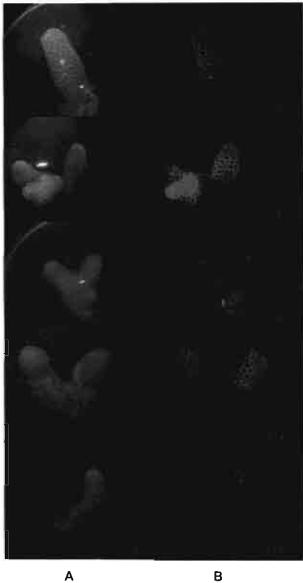
Figura 29. Fotografías de Porites divaricata empleando una lámpara azul y filtro amarillo expuestos a benzo[α]pireno, con radiación solar sin UV. (A) Radiación blanca; (B) radiación fluorescente. Los corales se observan blanqueados por exposición al hidrocarburo.
