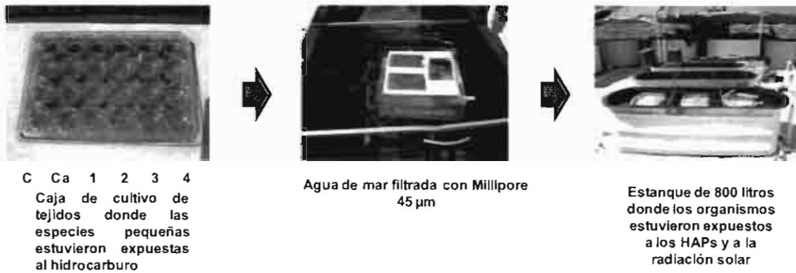
Figura 7. Diseño de pruebas experimentales para S. gigas y C. radiatum C=control de manipulación agua marina, Ca= Control con solvente (Acetona), 1, 2, 3, 4= Concentraciones nominales del hidrocarburo aromático policíclico (fluoranteno o benzo[ \alpha ]pireno).
