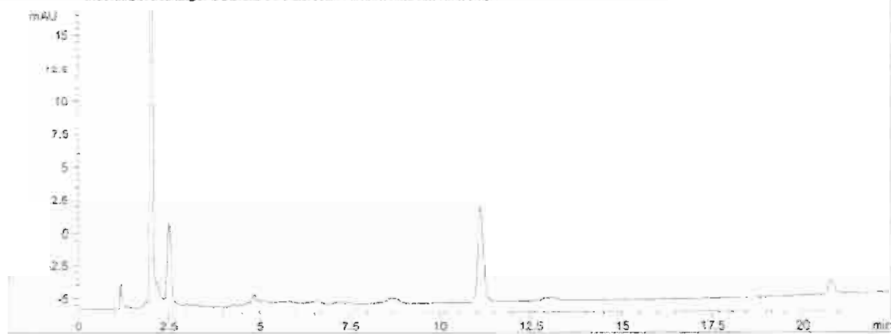
WVD1 A, Wavelength=230 nm, TT (MARZO2~1\0308538\538PAH35.D)
