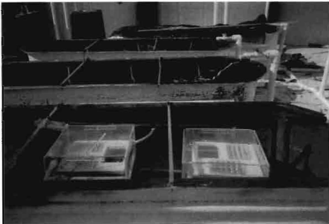
Figura 5. Bioensayos de larvas de S. gigas expuestas a fluoranteno y BAP, en placas de cultivo de tejidos cubiertas con placas de plexiglás.
