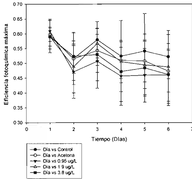
Figura 26. Eficiencia fotoquímica máxima del coral Porites divaricata expuestos a benzo[ \alpha ]pireno con radiación solar sin UV.
