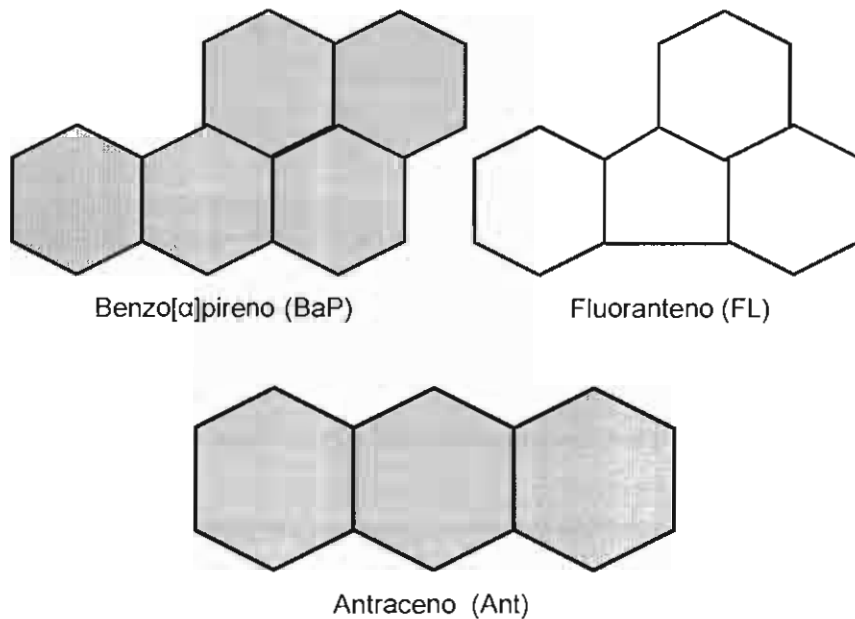
Figura 1. Estructura química de los hidrocarburos aromáticos policíclicos: Benzo[ \alpha ]pireno (BaP), Fluoranteno (FL) y Antraceno (Ant). Empleados en el presente trabajo.
