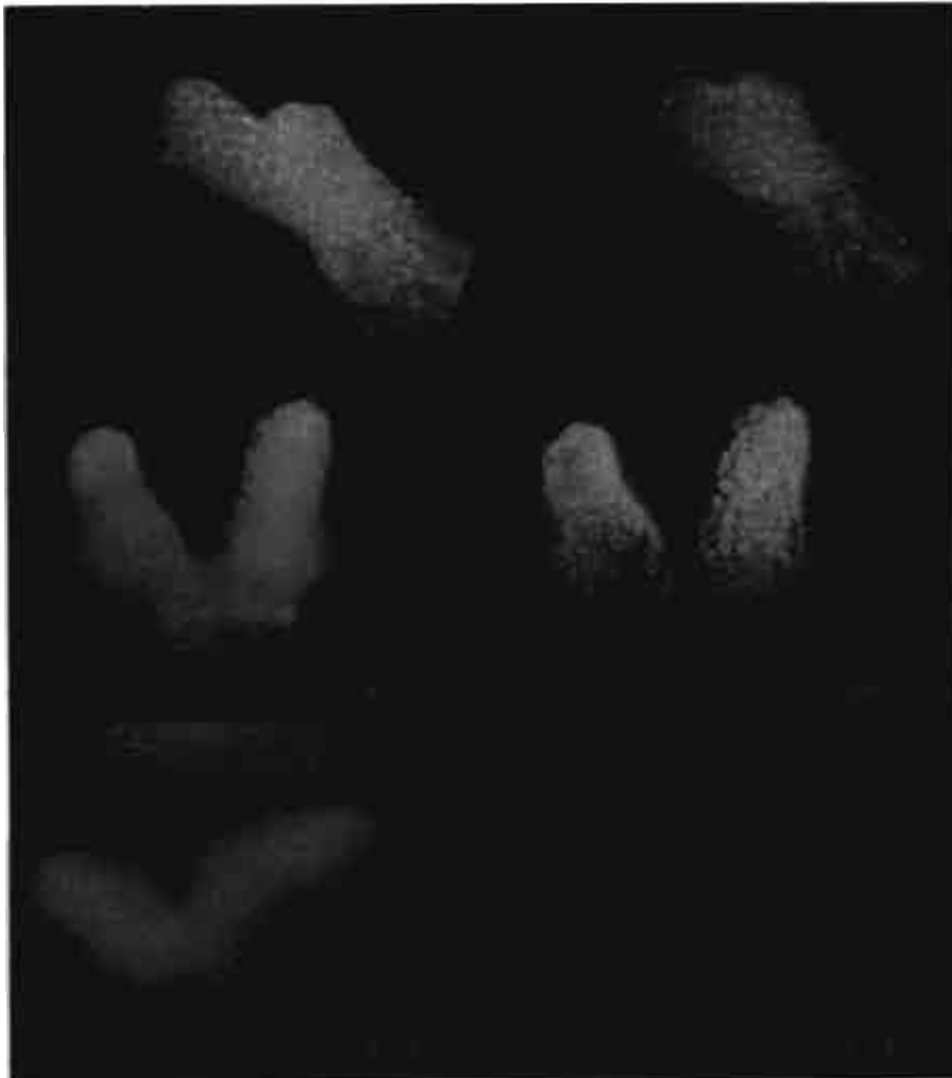
Figura 14. Porites divaricata expuesto al hidrocarburo, se identifican las diferentes etapas. (A) Radiación blanca; (B) Radiación fluorescente.
