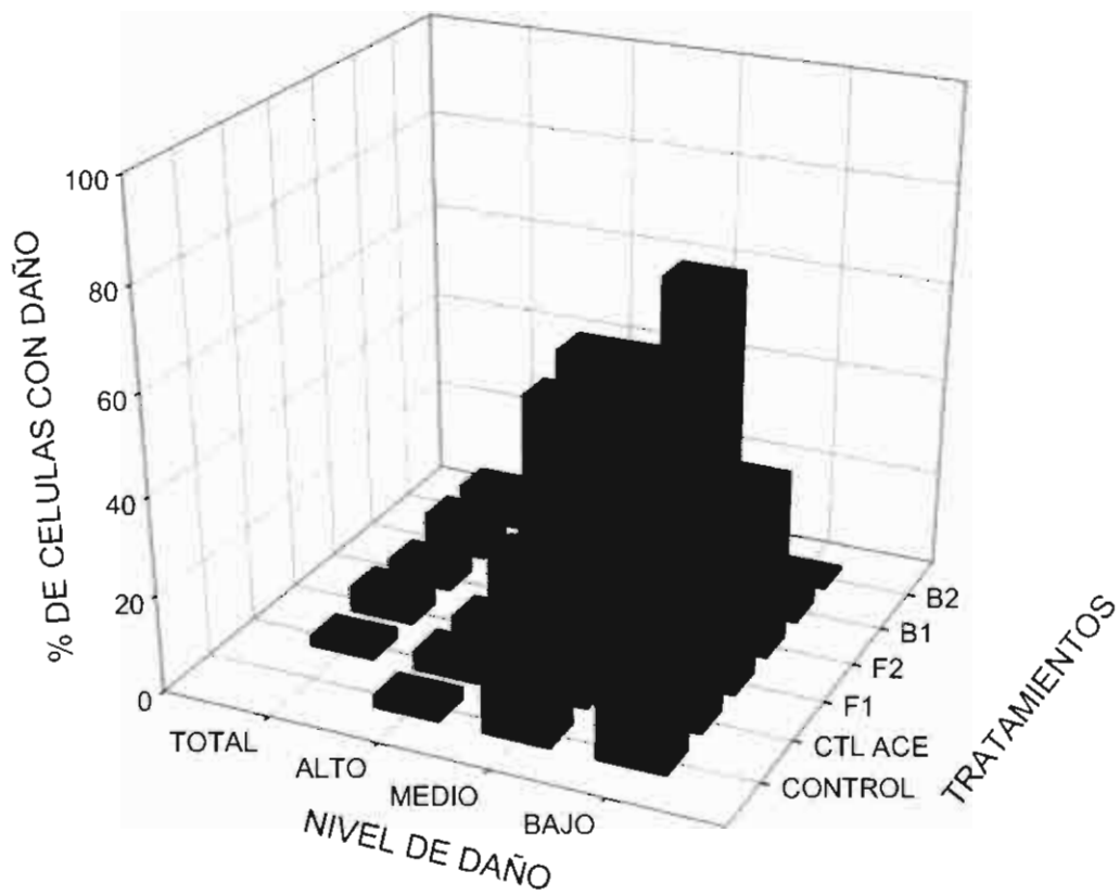
Figura 17. Respuesta de los metanauplios de A. franciscana expuestos a fluoranteno (F) benzo[ \alpha ]pireno (B). Datos compilados de más de 200 células. CTL ACE = control de acetona; F1= fluoranteno a 24 \mu\text{g/L} ; F2= fluoranteno a 48 \mu\text{g/L} ; B1= benzo[ \alpha ]pireno a 4.8 \mu\text{g/L} ; B2= benzo[ \alpha ]pireno a 9.6 \mu\text{g/L} .
