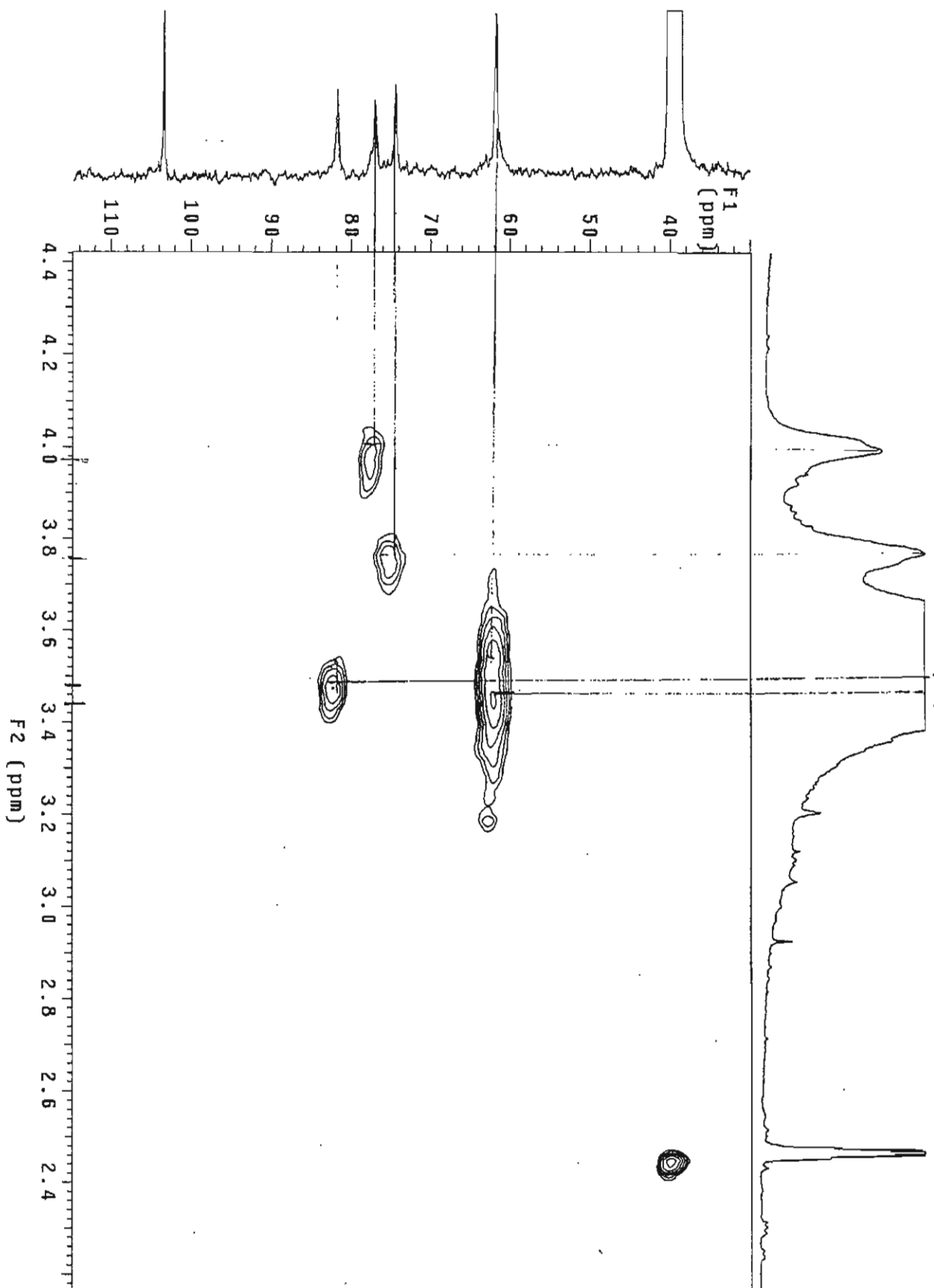
Figura 8. Espectro de HETCOR de la peltalosa
