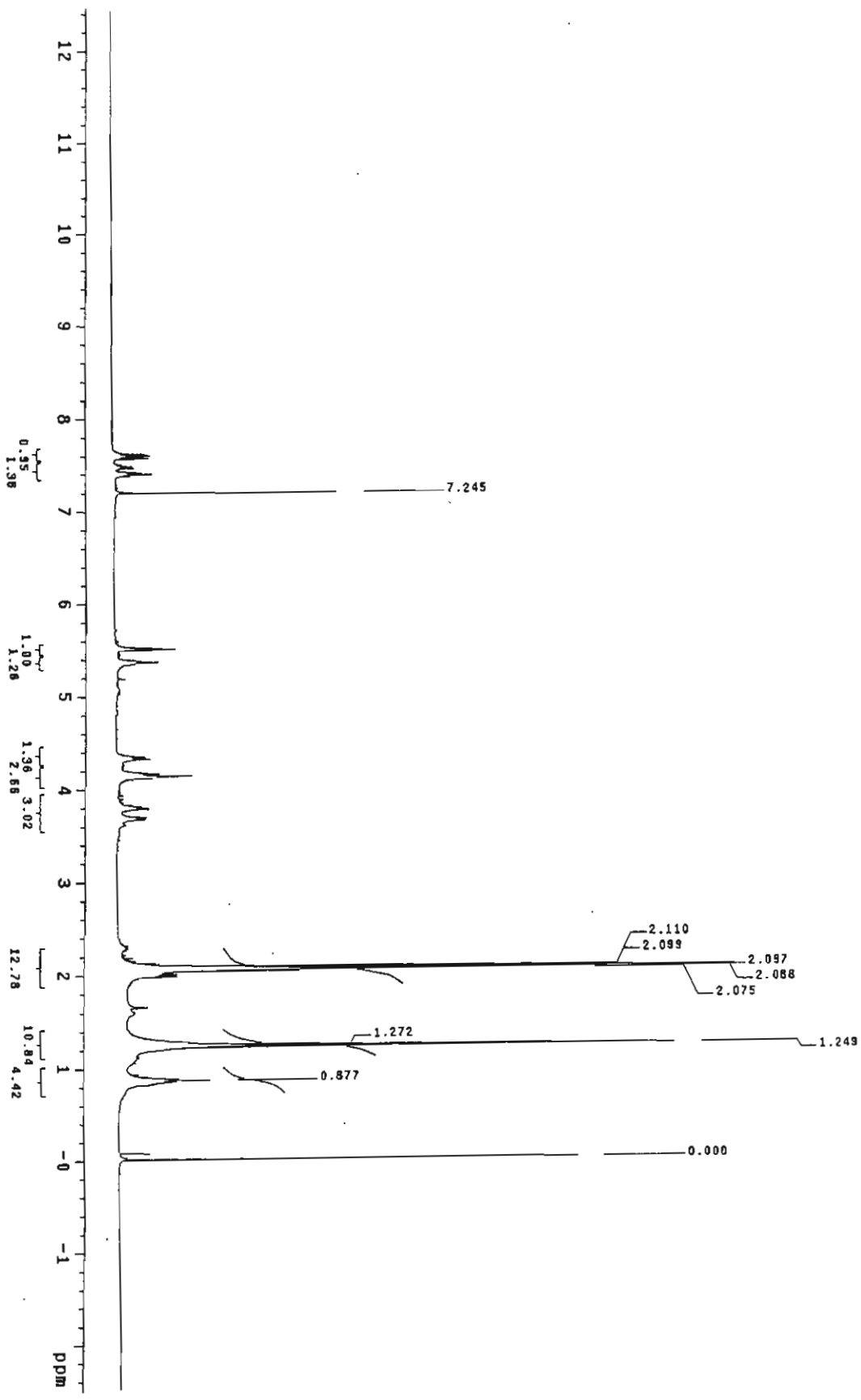
Figura 10. Espectro de 1 H RMN del Acetato de Petalosa
