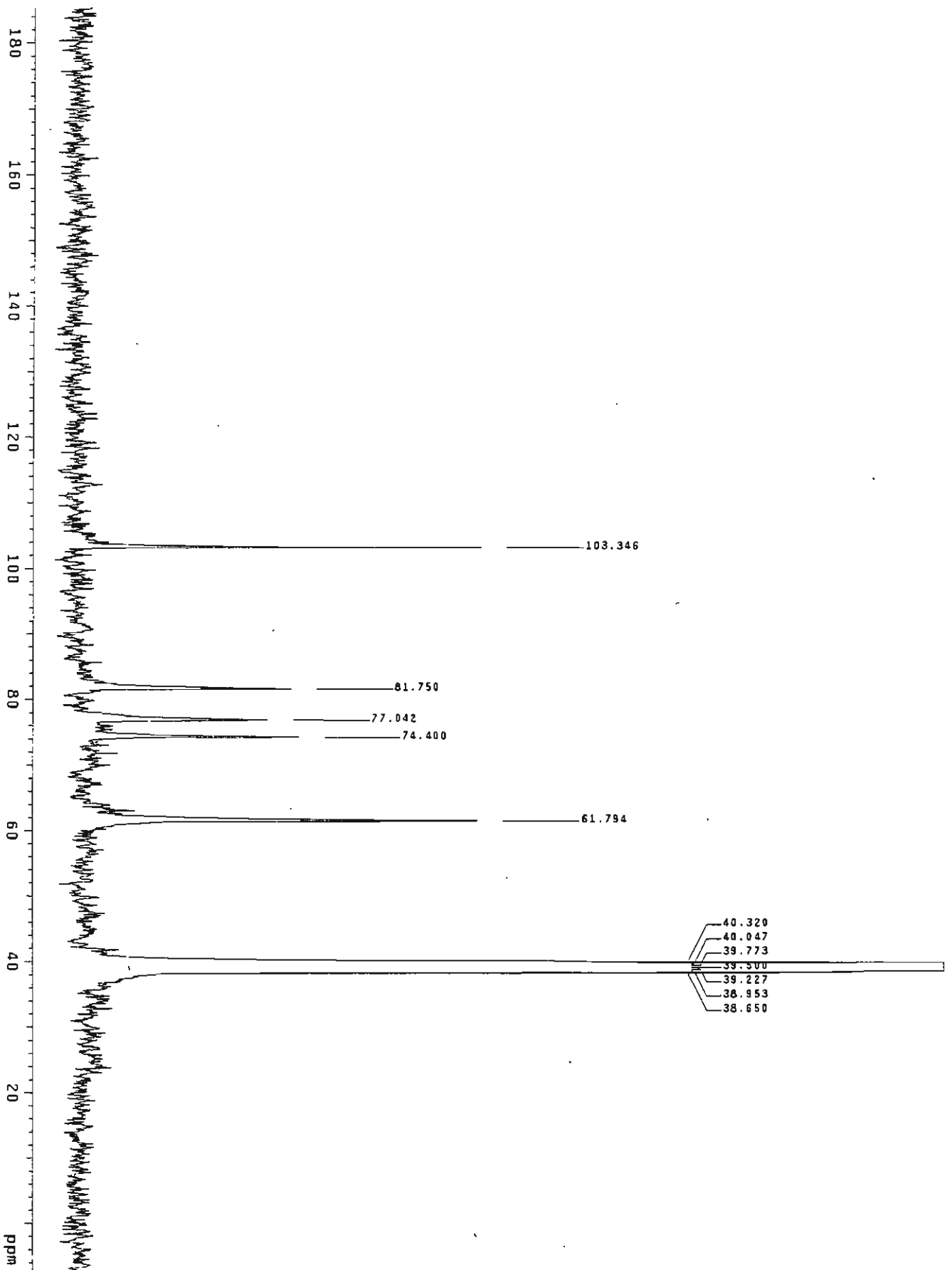
Figura 5. Espectro de ^{13}\text{C} RMN de la peltalosa
