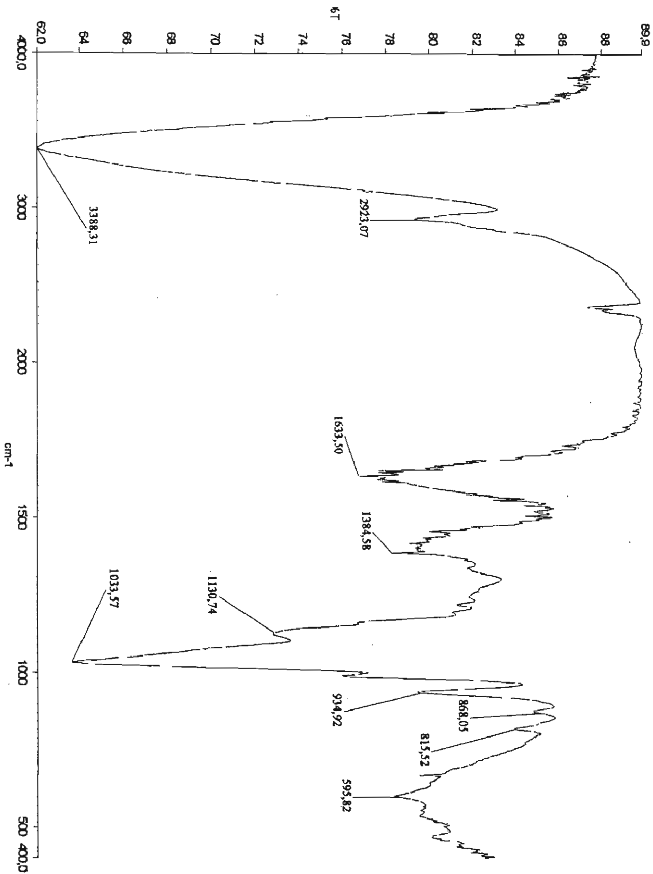
Figura 3. Espectro de IR de la peltalosa
