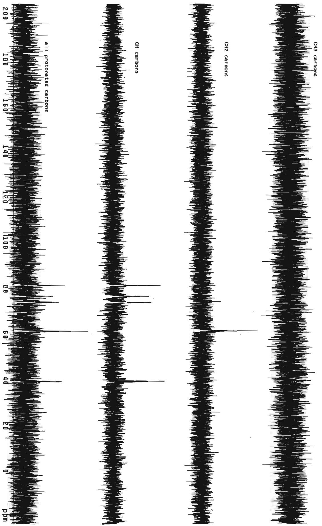
Figura 6. Espectro DEPT de la peltalosa
