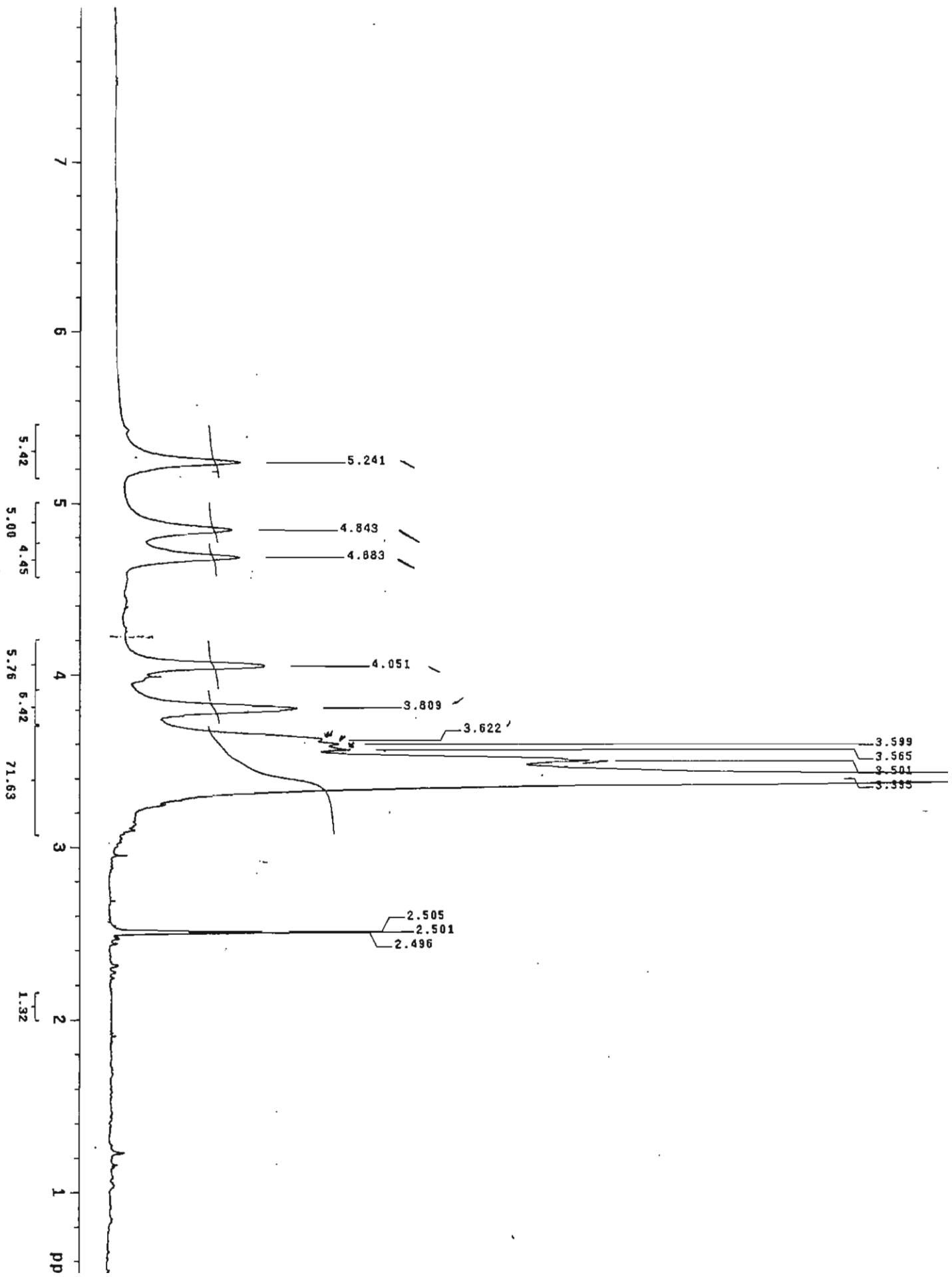
Figura 4. Espectro de ^1\text{H} RMN de la peltalosa
