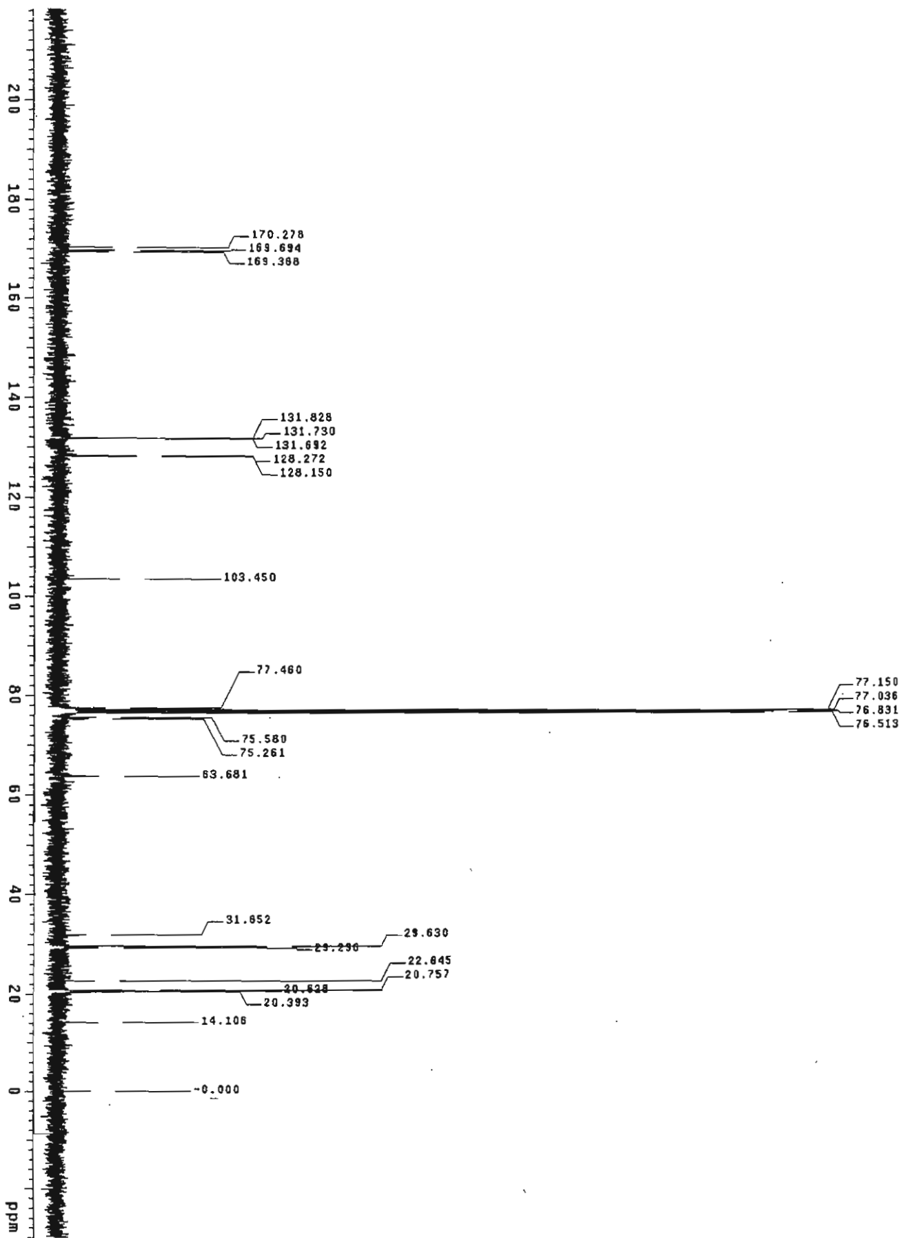
Figura 11. Espectro de ^{13}\text{C} RMN del Acetato de Peltalosa
