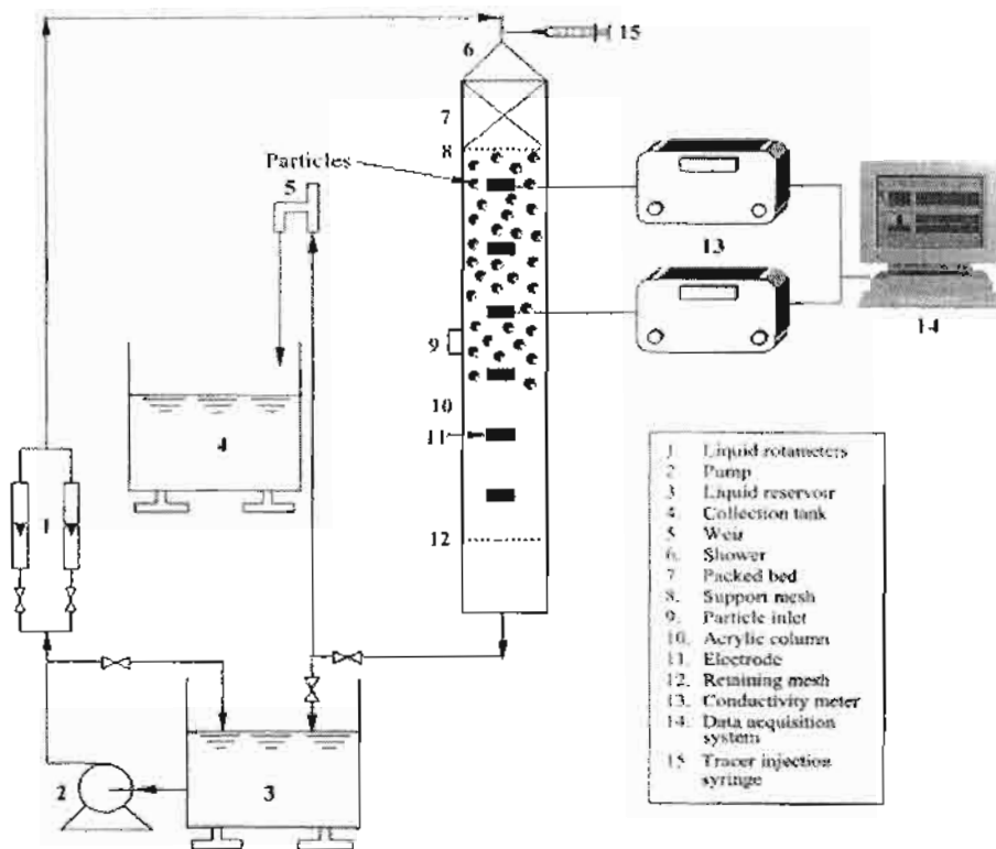
Fig 7 Reactor de lecho fluidificado inverso (LFI)*
