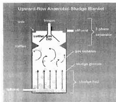
Fig. 6 Reactor de lecho de lodos de flujo ascendente (UASB)*.
